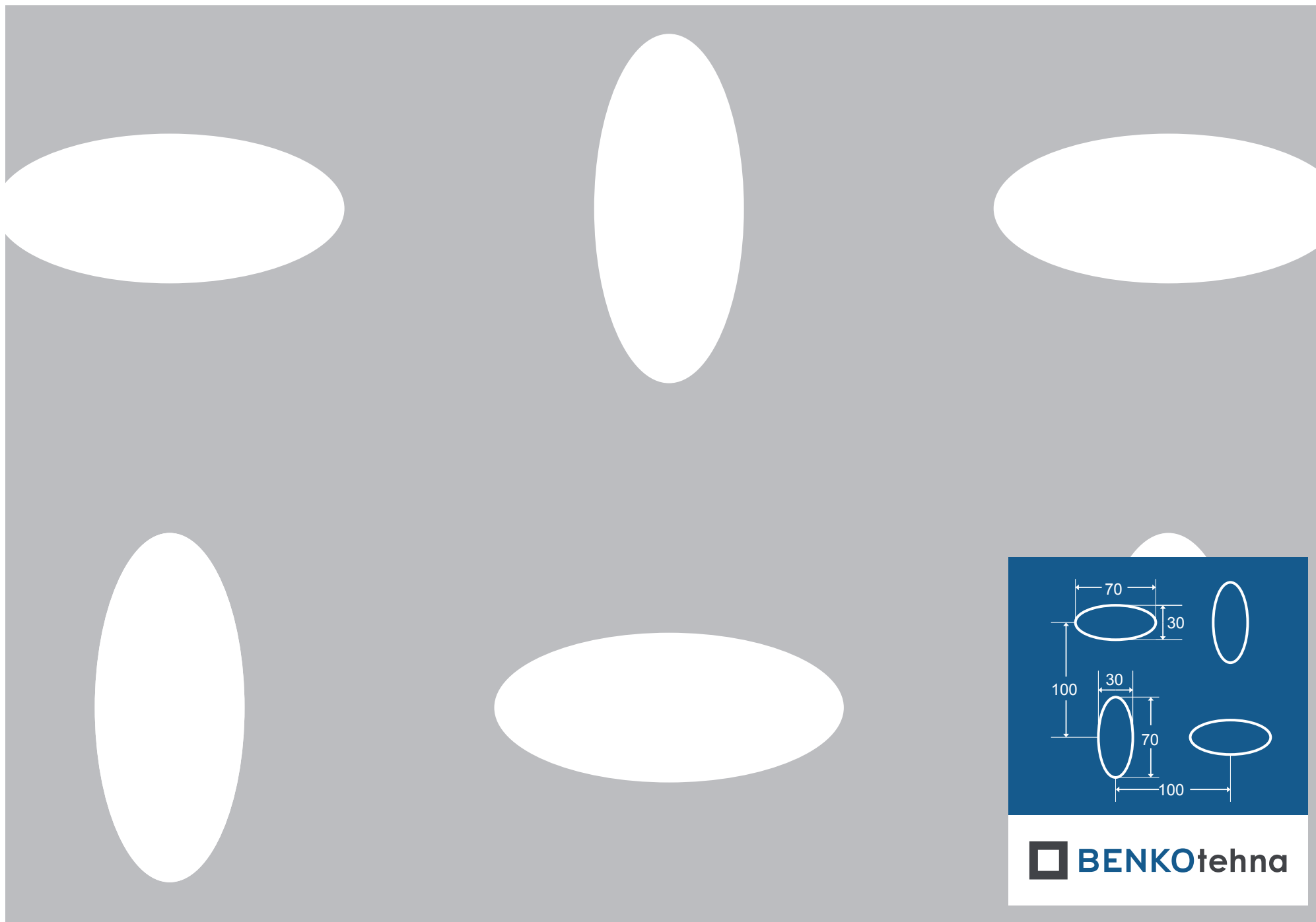
CL - EVH 30×70/100×100: otvorenost = 16,5%
