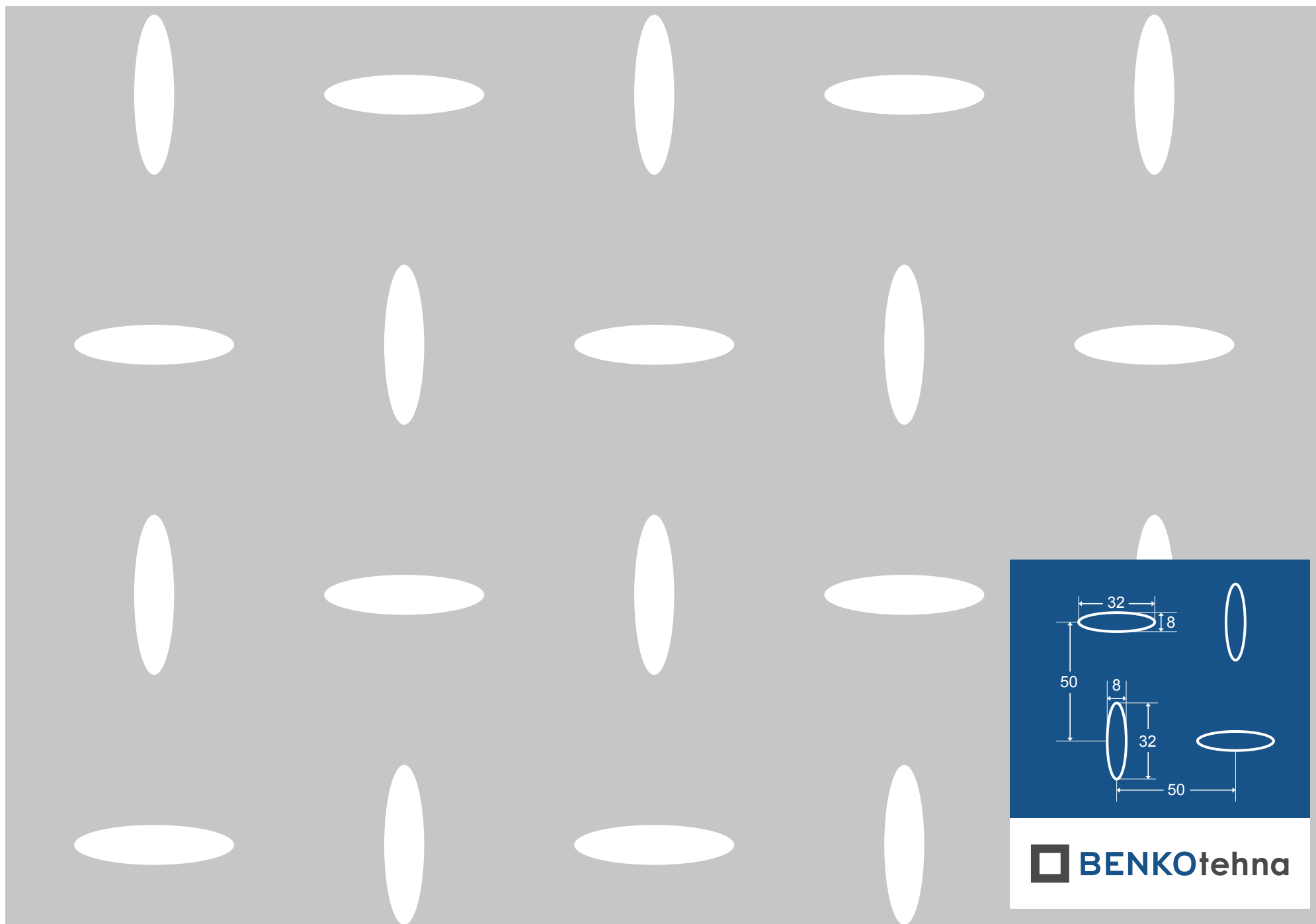
CL - EVH 8×32/50×50: otvorenost = 8,0%
